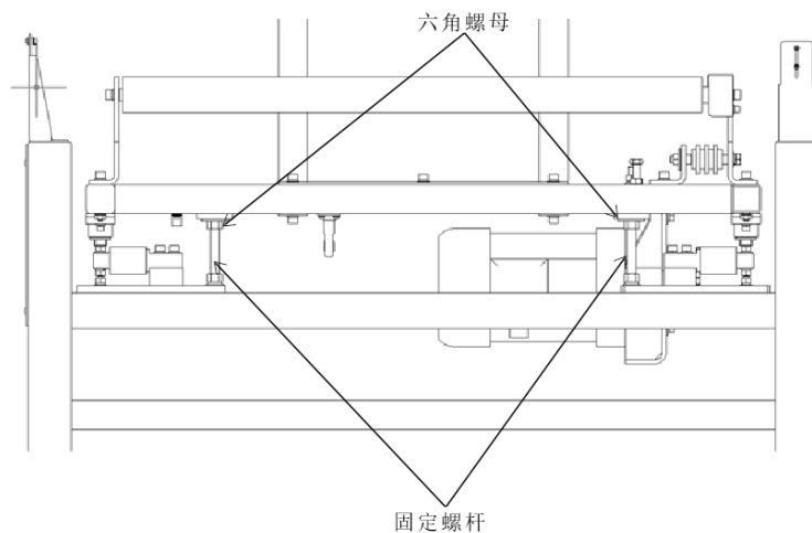
图 3-2 限位位置
