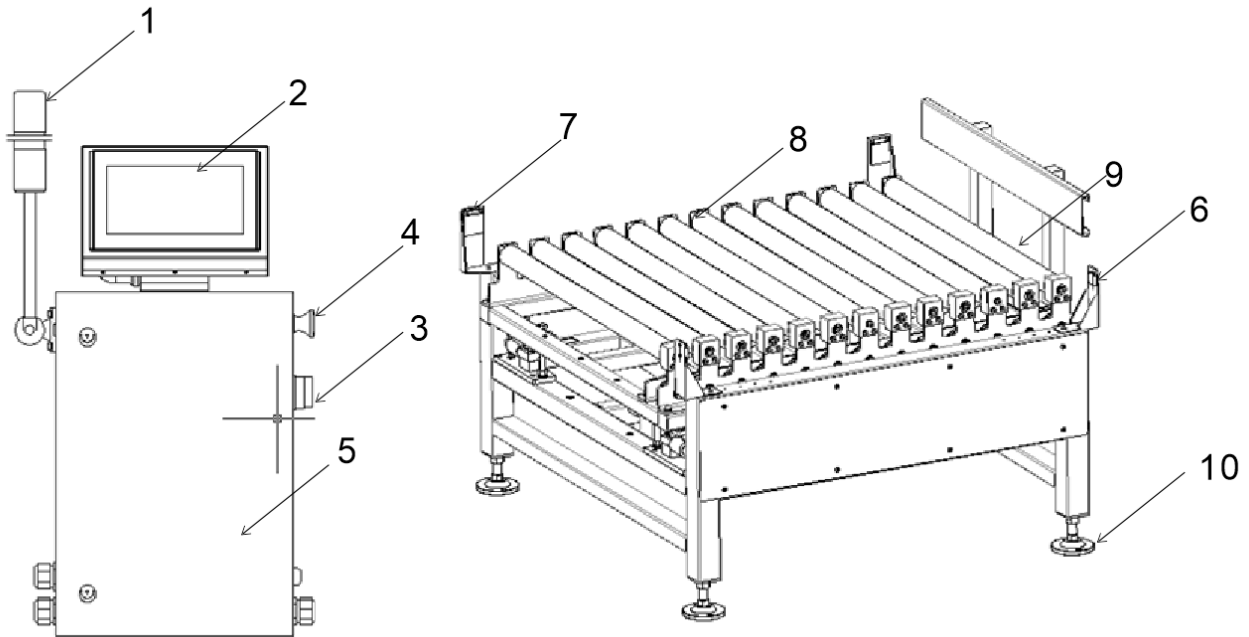
图 2-1 整体外观
