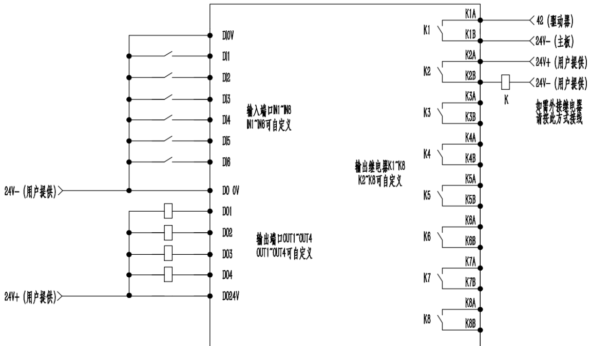
图 2-3 入输出口接线示意图
